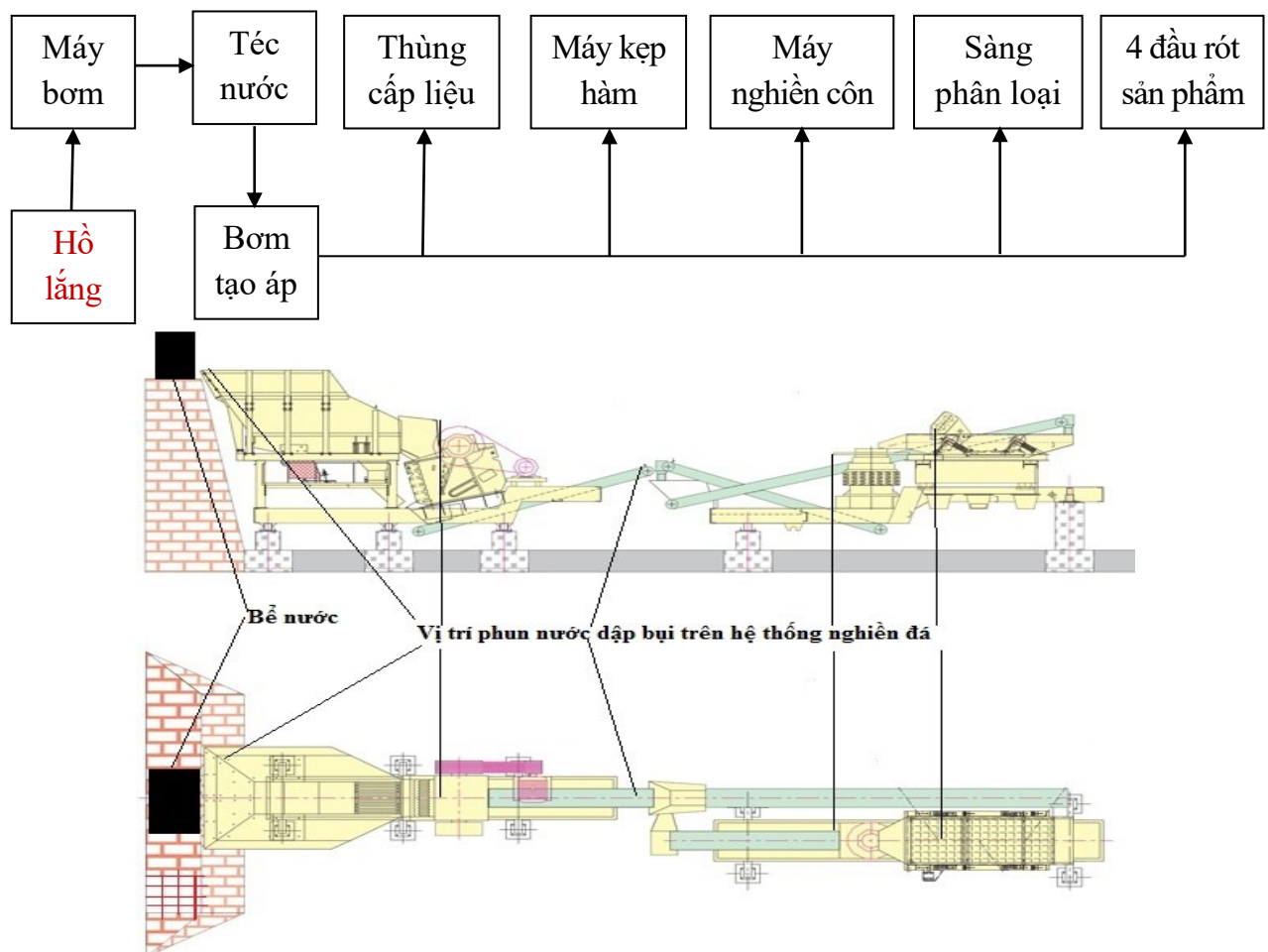
Hình 3.3: Sơ đồ nguyên lý cấp nước chống bụi dây chuyền nghiền sàng
